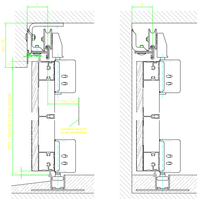
Sturzbereich
