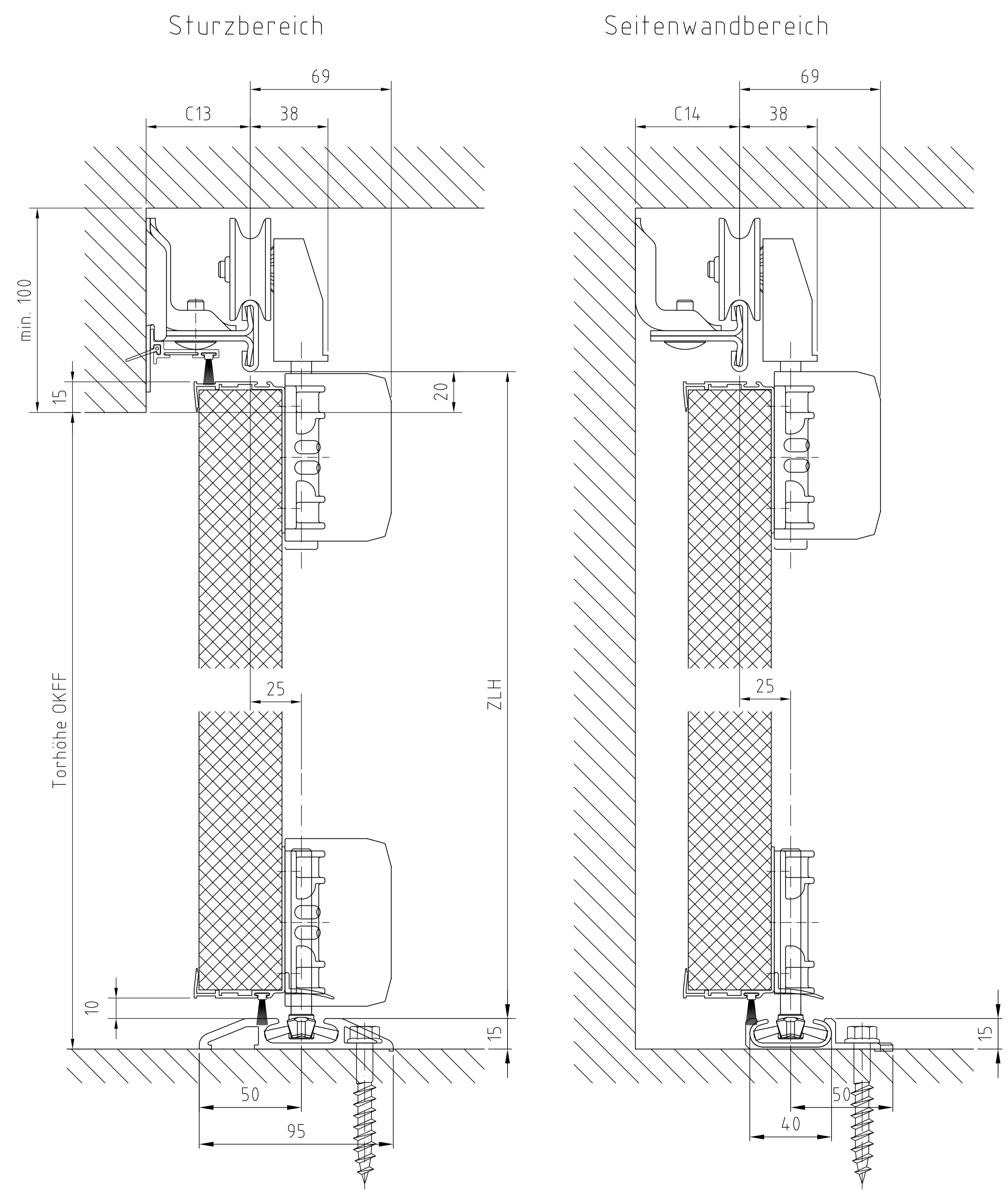
mit Alu-Renovations-Bodenschiene
