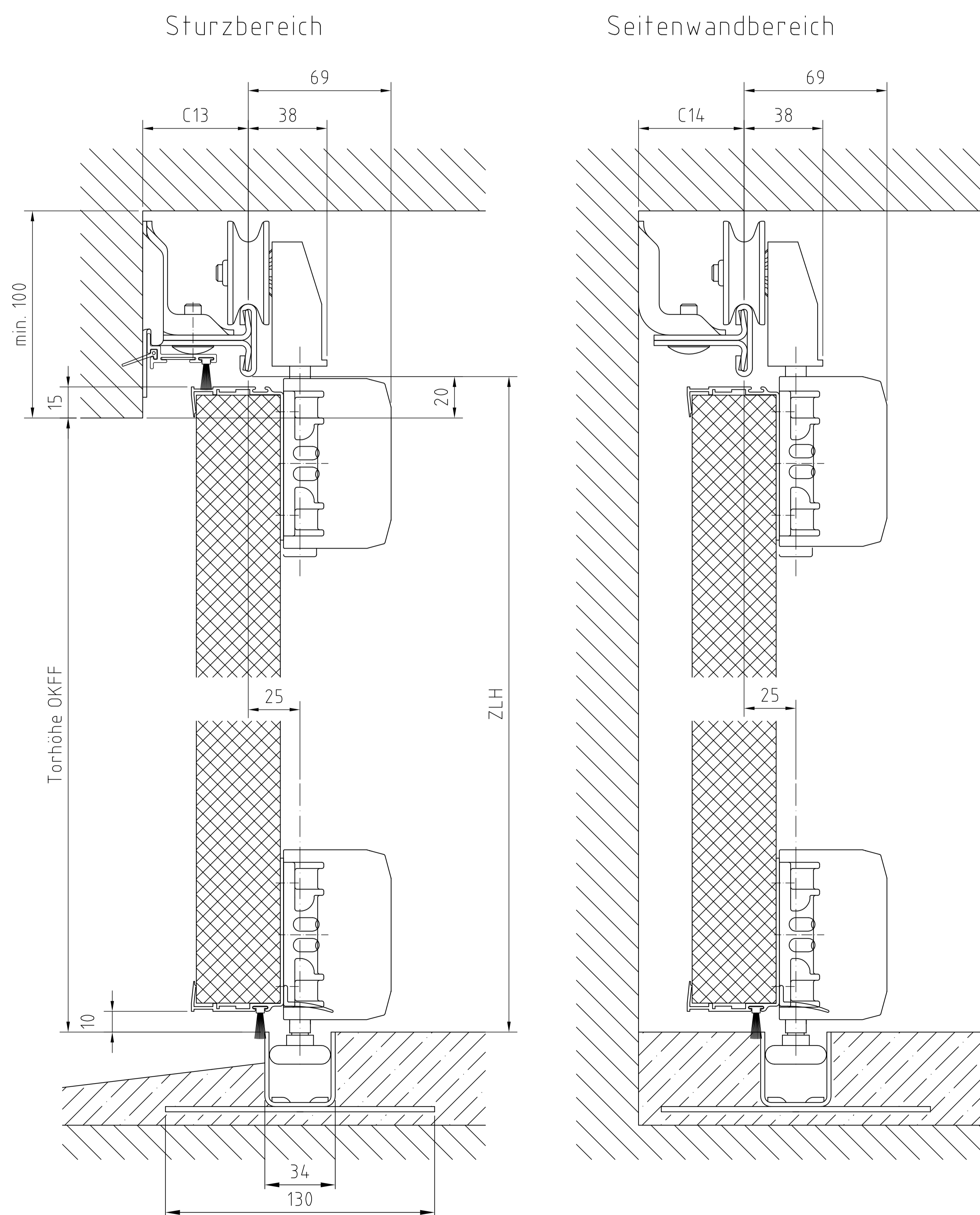
mit Normal-Bodenschiene
